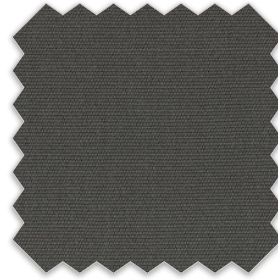
R-198 - NICKEL
